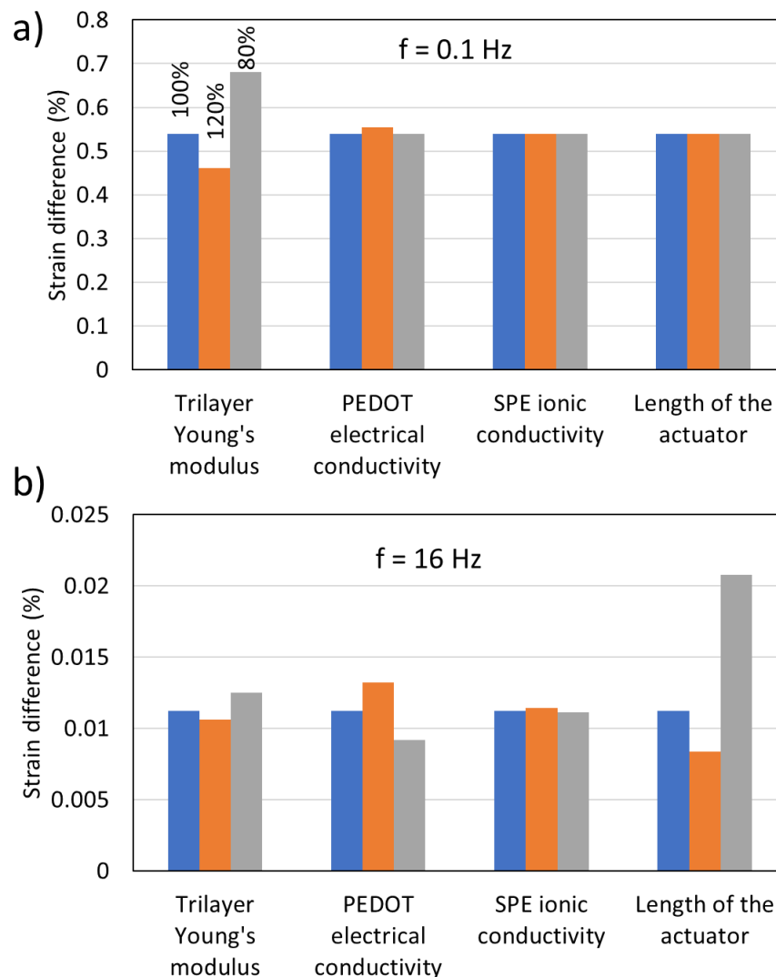
Fig.7 Facteurs clés affectant le déplacement de l'actionneur sous une tension carrée ( V_{pp} = 2,4 V), a) à basse fréquence f = 0,1 Hz, et b) à haute fréquence f = 16 Hz. Pour chaque paramètre il y a trois colonnes qui, de gauche à droite représentent la valeur réelle (colonne bleue), l'effet lorsque la valeur est augmentée de 20% (colonne orange) et l'effet lorsque la valeur est réduite de 20% (colonne grise).
